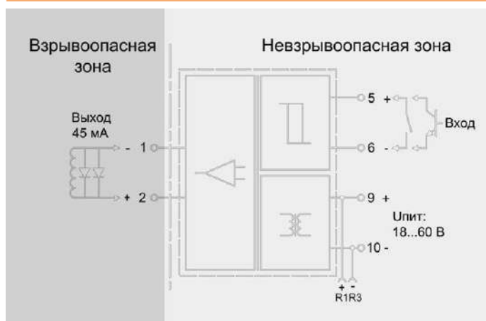
Схема выходной цепи
